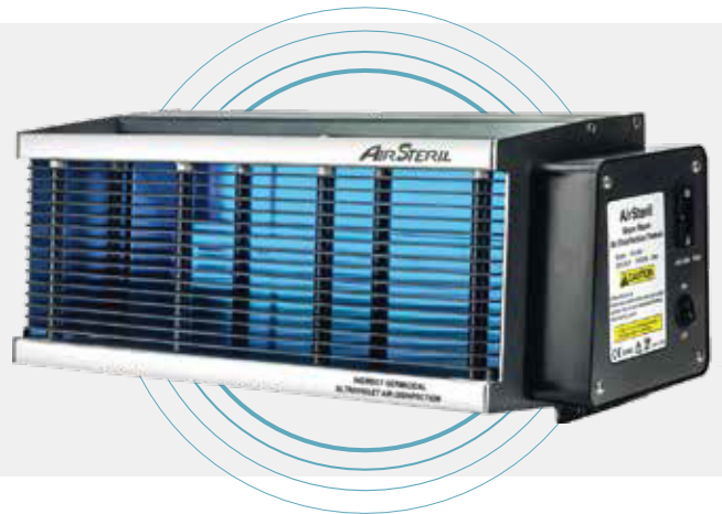
UPPER ROOM UVGI : 460mm (l) x 186mm (w) x 186mm (d) เครื่องเจือจางเชื้อโรคในอากาศ
