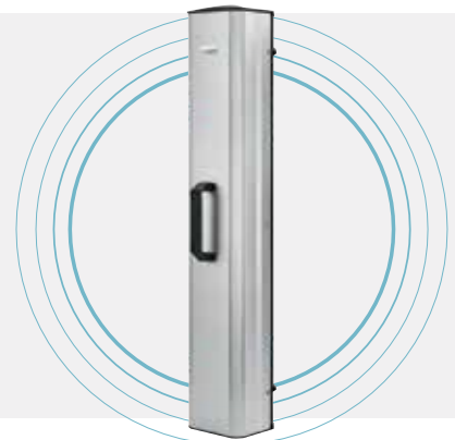
MP100 : 750mm (l) x 130mm (w) x 100mm (d)
